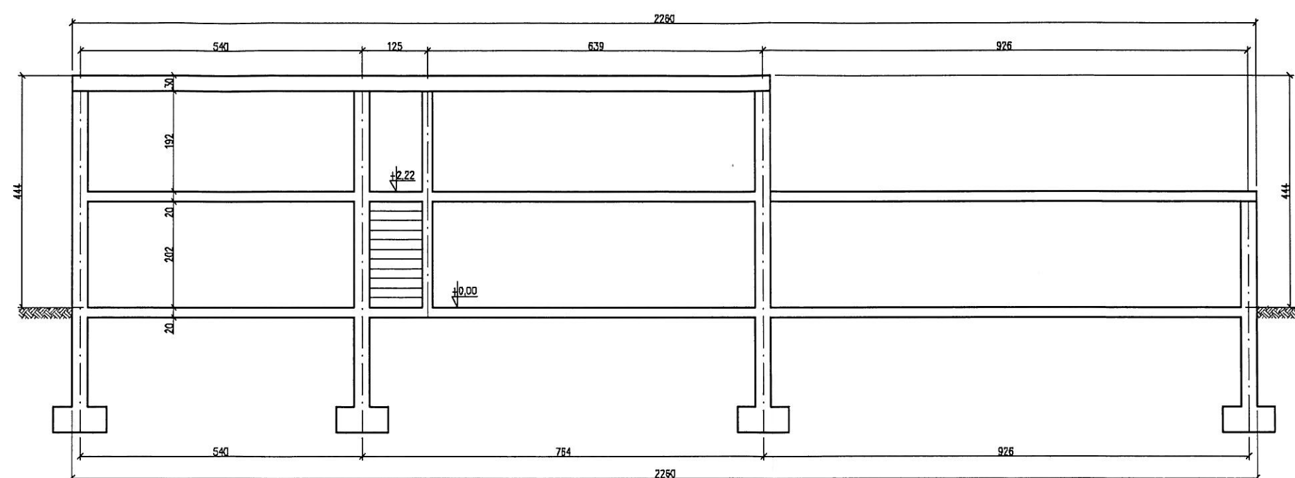
PRZEKRÓJ POPRZECZNY A-A
