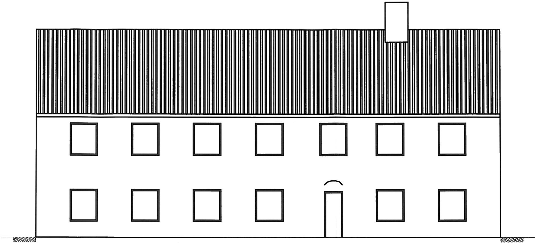
ELEWACJA FRONTOWA
