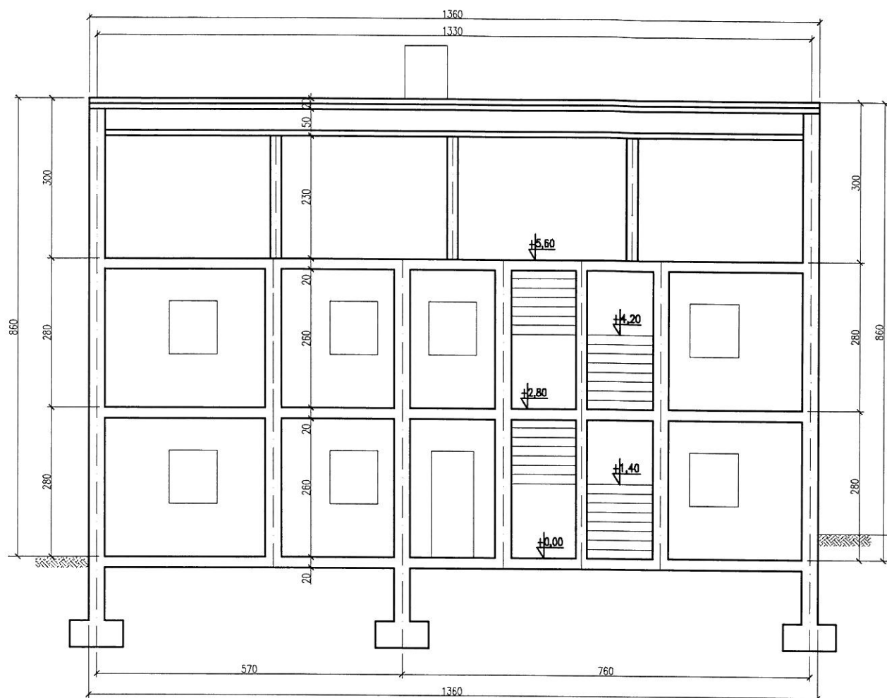
PRZEKRÓJ POPRZECZNY A-A
