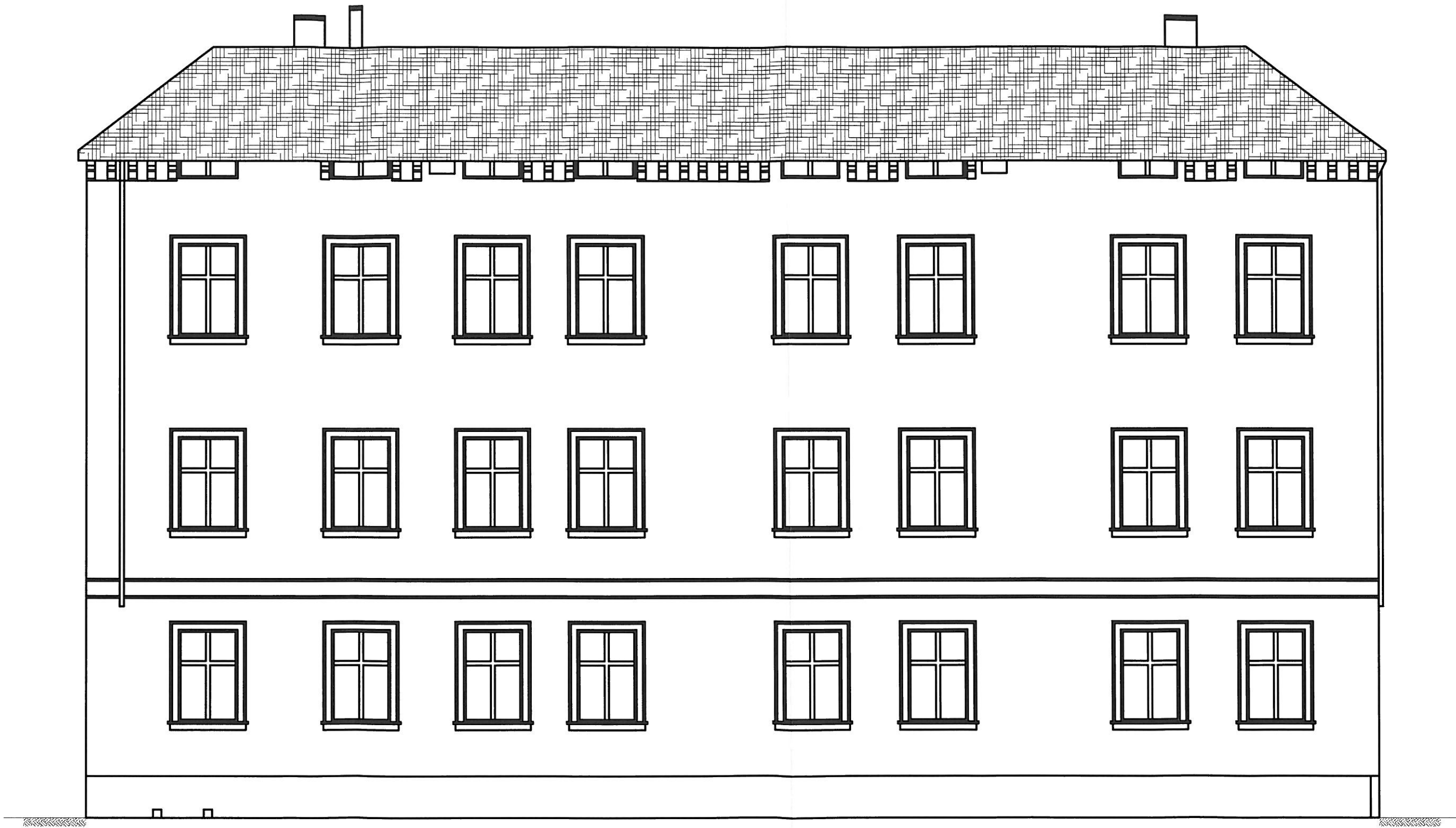
ELEWACJA BOCZNA - LEWA
