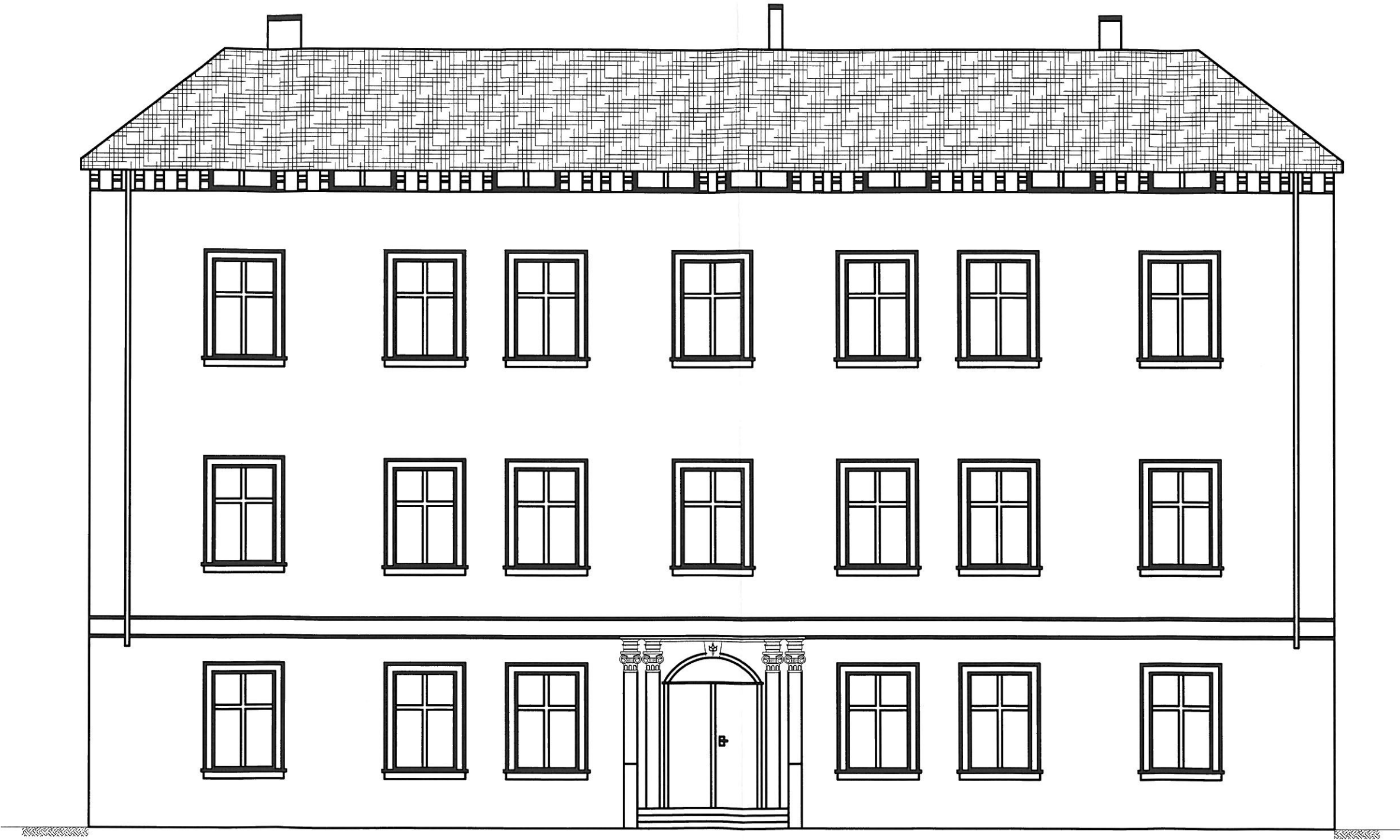
ELEWACJA FRONTOWA
