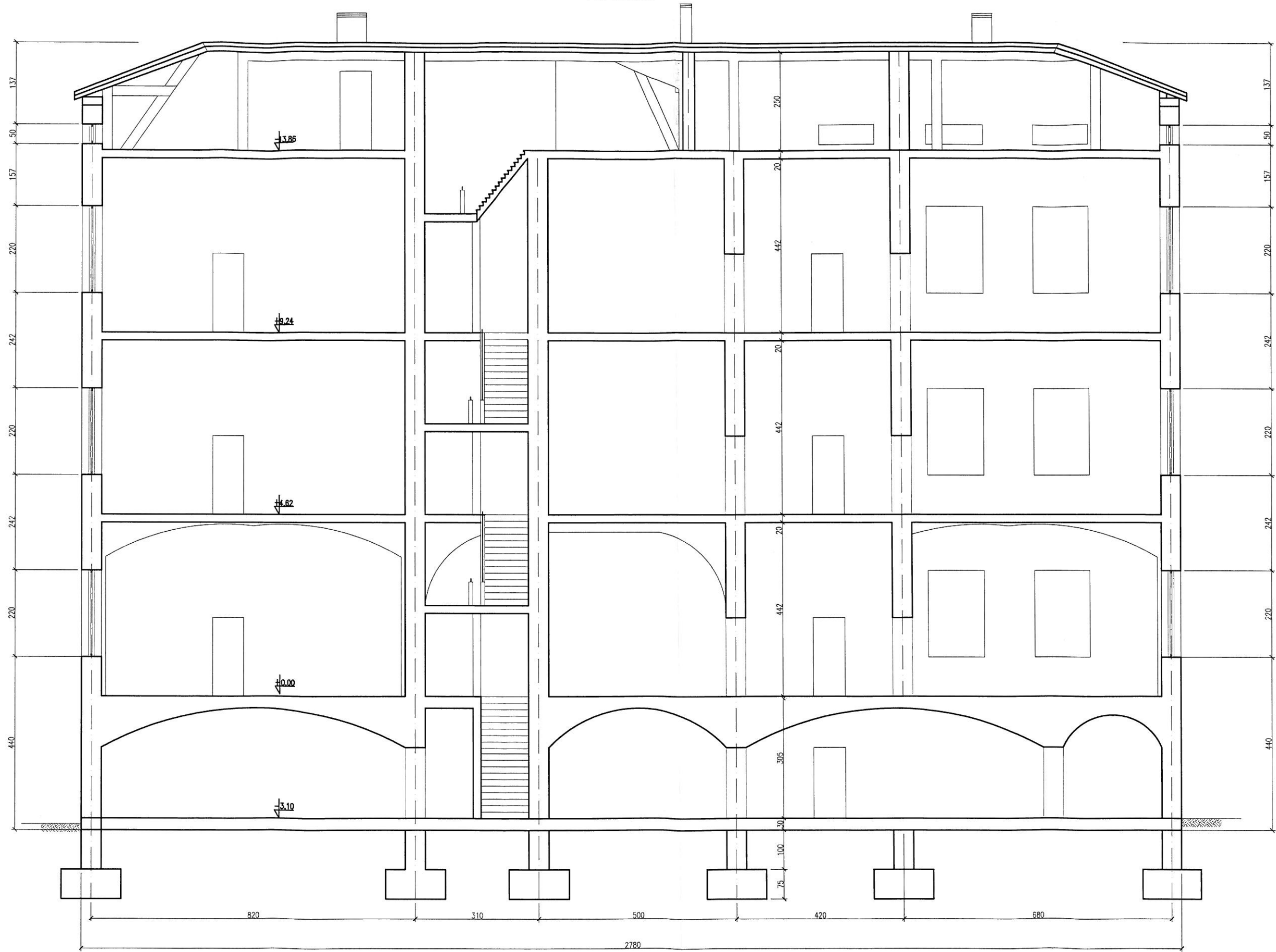
PRZEKRÓJ POPRZECZNY A-A
