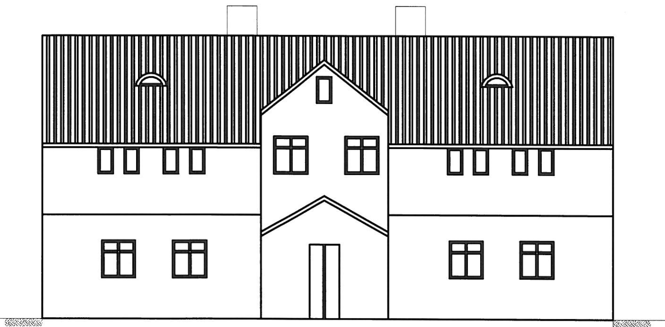
ELEWACJA FRONTOWA
