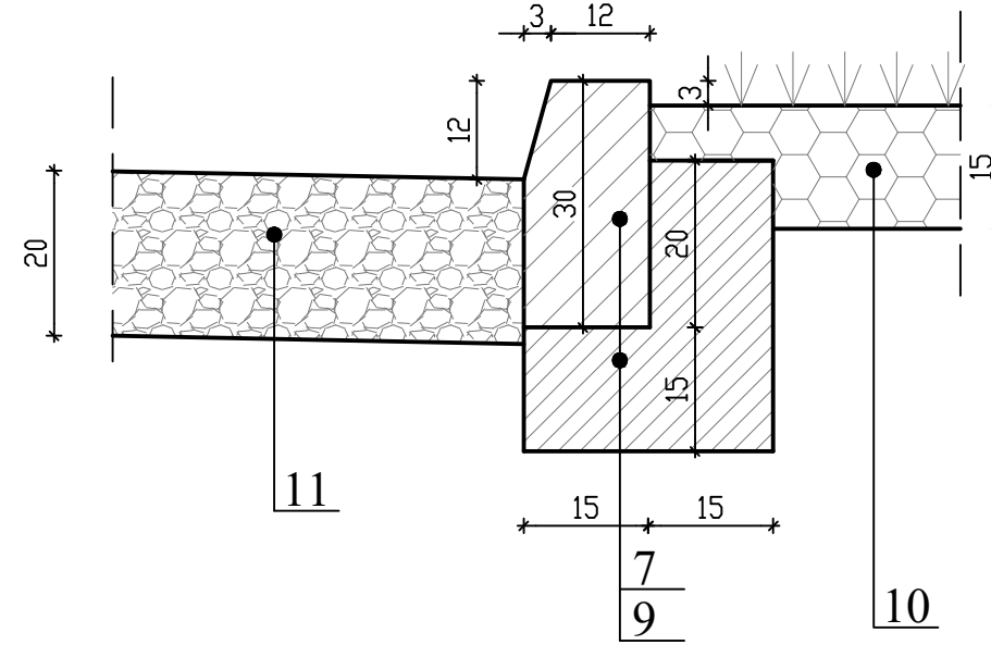
REMONTOWANA JEZDNI TŁUCZNIOWA ZIELEŃ
