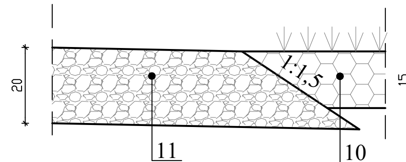
REMONTOWANA JEZDNI TŁUCZNIOWA ZIELEŃ
