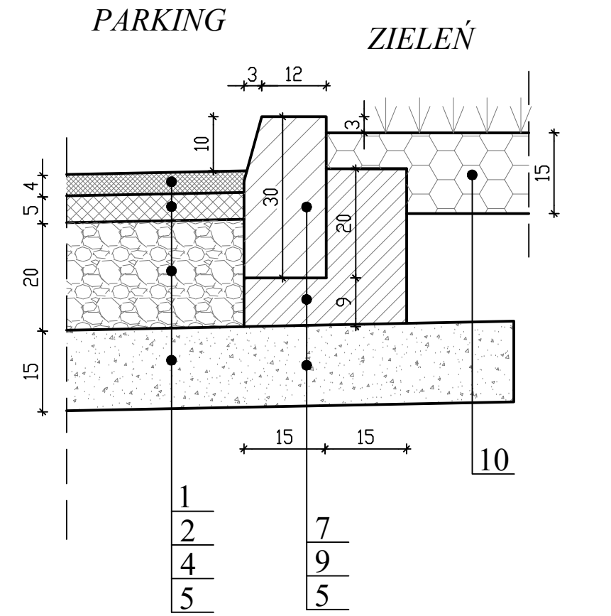
REMONTOWANA JEZDNI TŁUCZNIOWA
