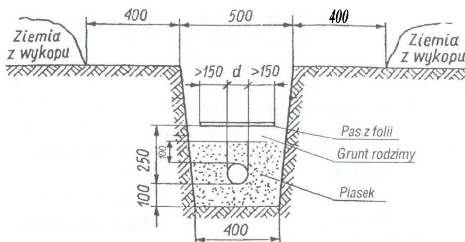
Rys. 1 Sposób układaniu kabli w ziemi
